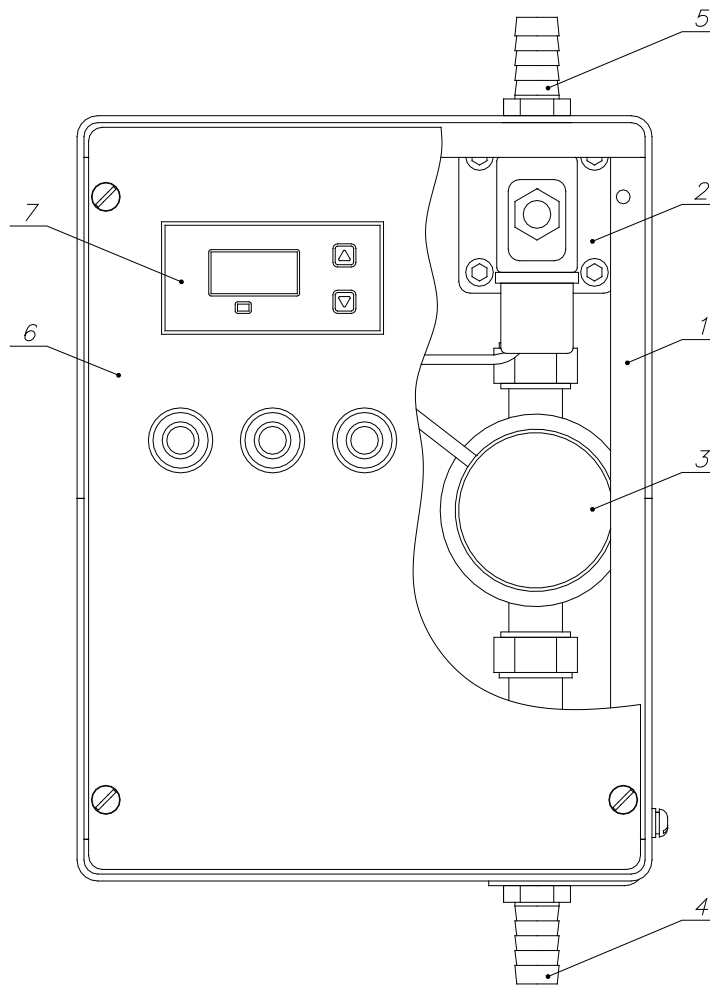
Рисунок 2. Дозатор воды.
