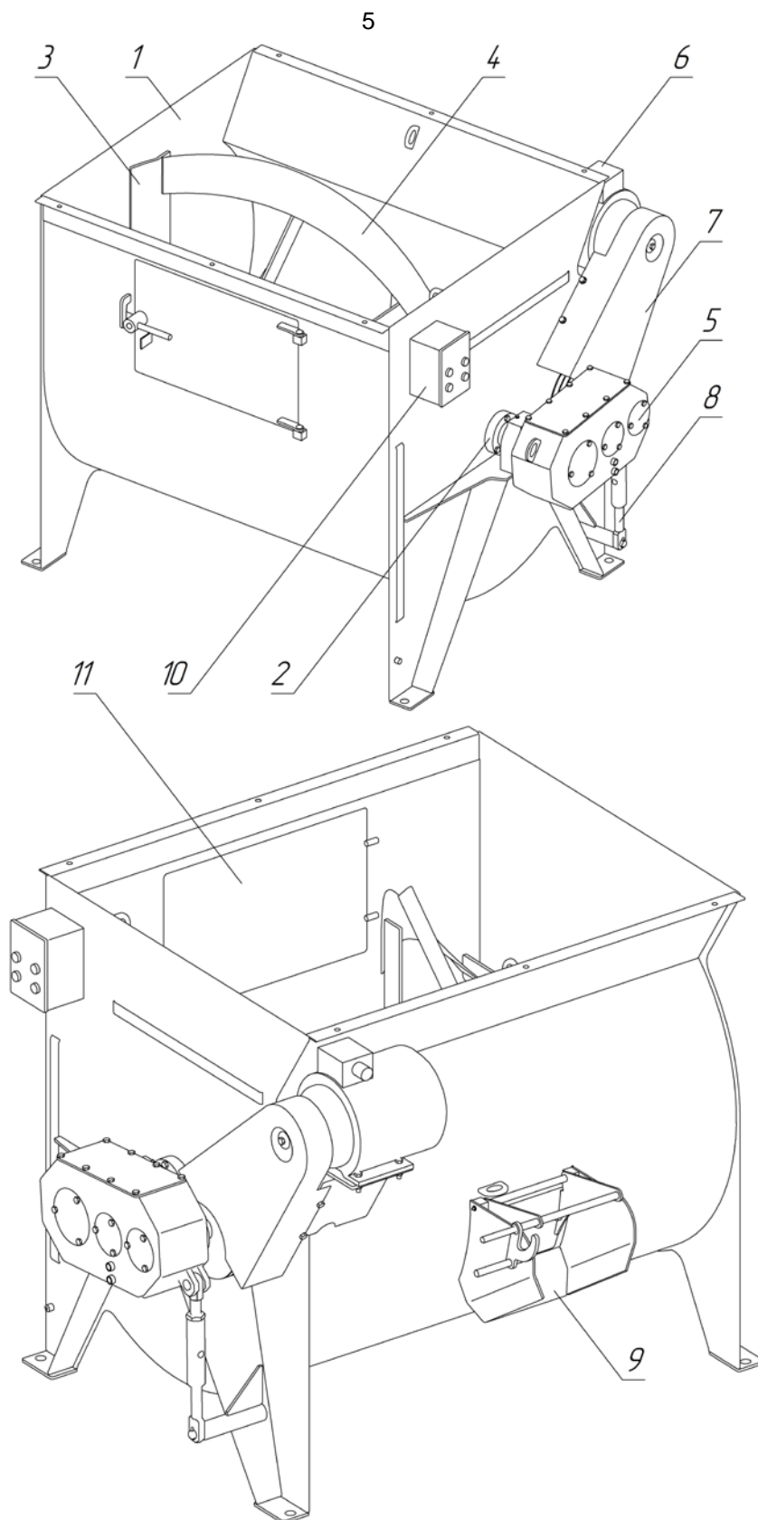
Рисунок 1. Смеситель СГ-1000-А.
