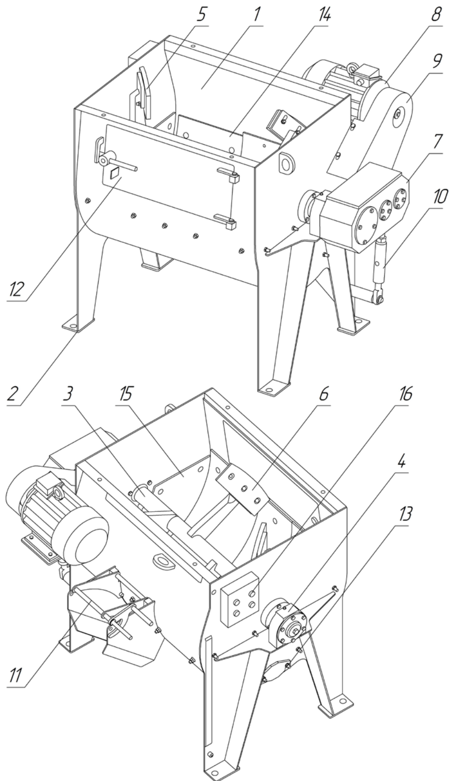
Рисунок 4. Смеситель СГ-350.
