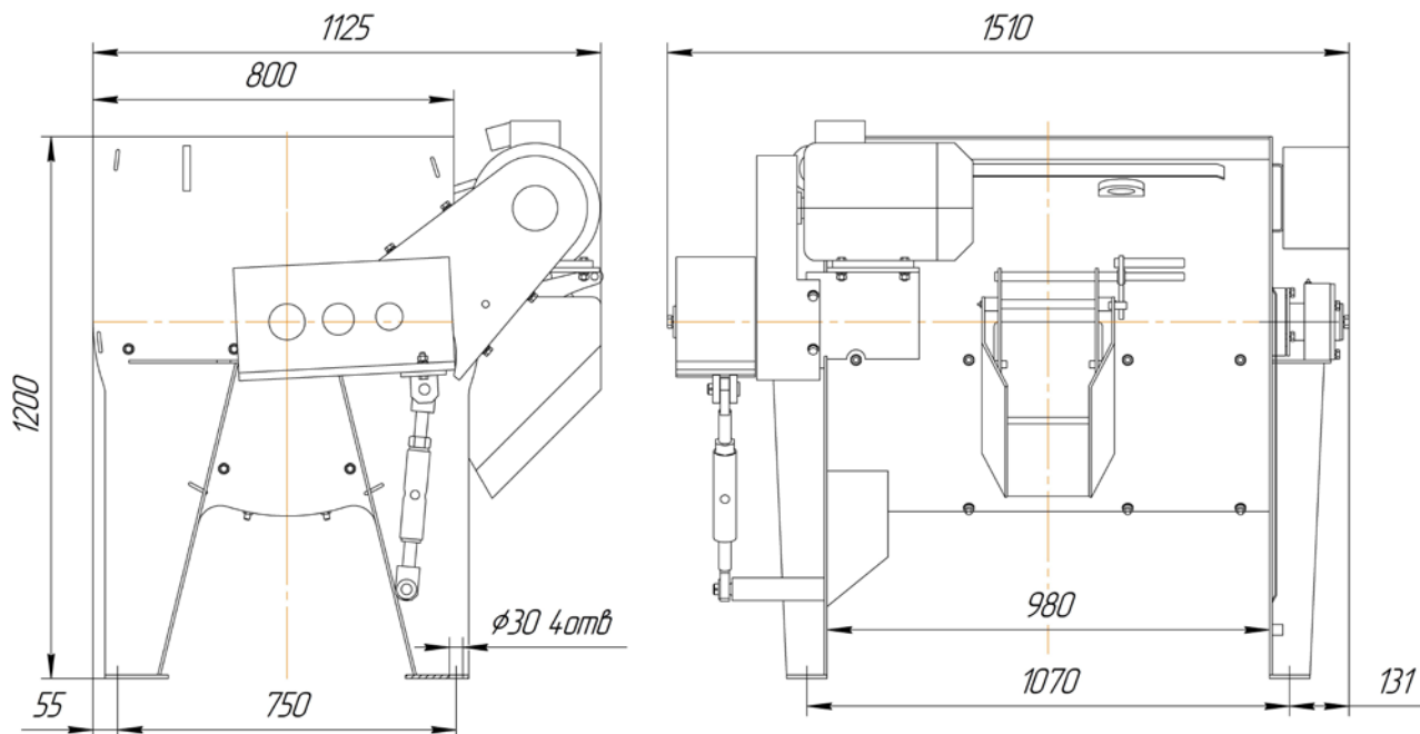
Рисунок 5. Габаритно-присоединительные размеры СГ-350.
