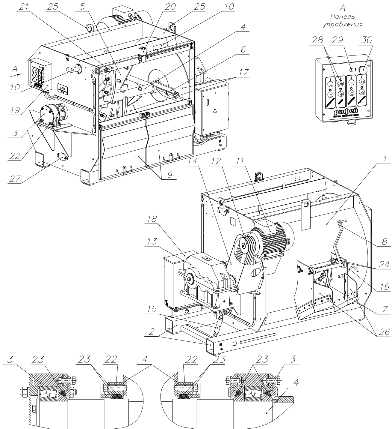
Рис. 3. Смеситель.
